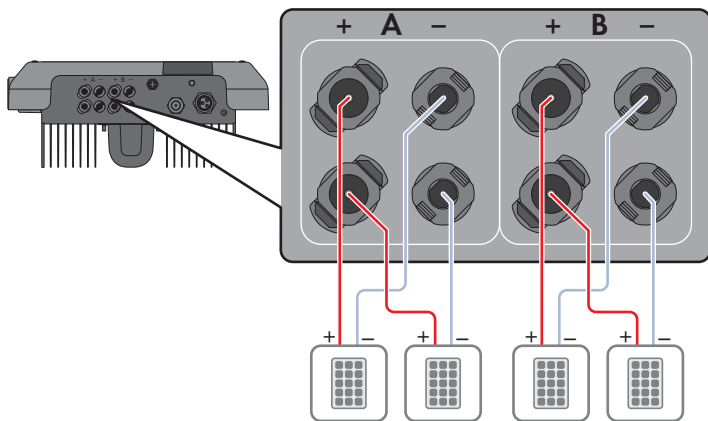
Figura 10: Panoramica del collegamento nel funzionamento normale
